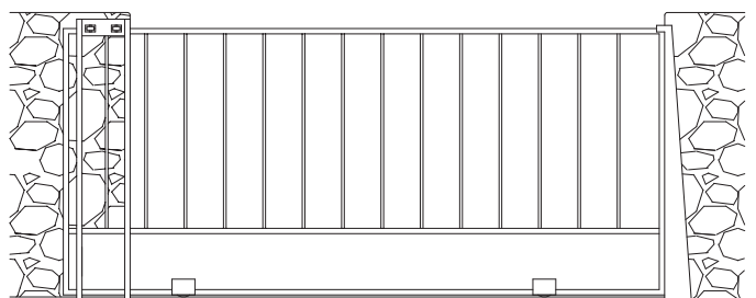
ALZADO
